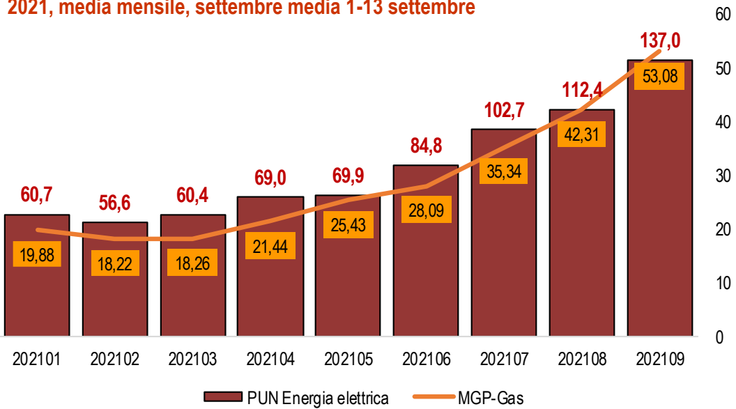
Energia elettrica - Prezzo d'acquisto. PUN (€/MWh) e prezzi del gas-mercato giorno prima 2021, media mensile, settembre media 1-13 settembre
